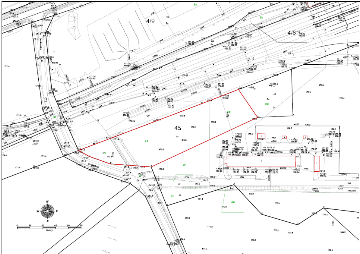
Rysunek 1 – rzut działki 45/ SITE No 45
